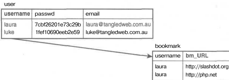
РИСУНОК 24.2 Схема базы данных для системы RHPBookmark.
