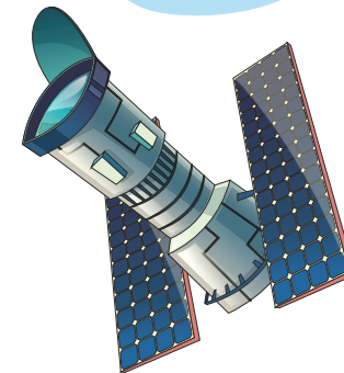
КОСМІЧНИЙ ТЕЛЕСКОП “ГАББЛ”
