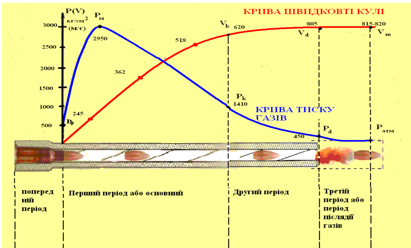
Мал. №1. P_f - тиск форсування; P_m – найбільший (максимальний) тиск; P_k та V_k – тиск газів і швидкість кулі в момент закінчення горіння пороху; P_d та V_d – тиск газів і швидкість кулі в момент вильоту кулі з каналу ствола; V_m – найбільша (максимальна) швидкість кулі; P_{атм} – тиск дорівнюючий атмосферному.
