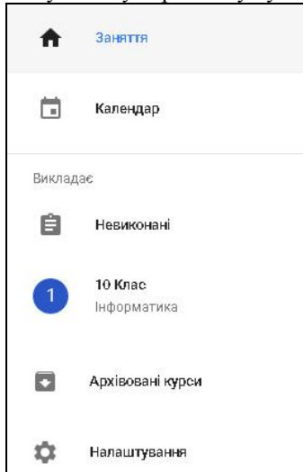
Рис. 7.2 Меню курсу
