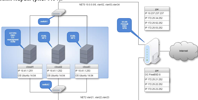
Рис. 9.14. Схема мережі розширеної зони.
