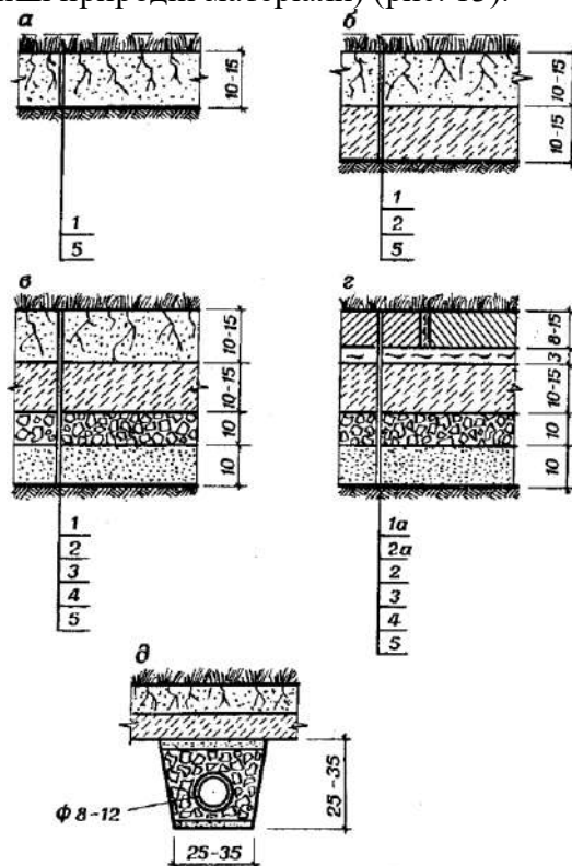
Рис. 13. Конструкція основи газону (а – одношарова, б – двошарова, в, г – багатошарова, д – дренаж): 1 – засівний шар (1а, 2а – компостні прошарки), 2, 4 – піщаний шар, 3 – щебневий шар, 5 – суглинок.
