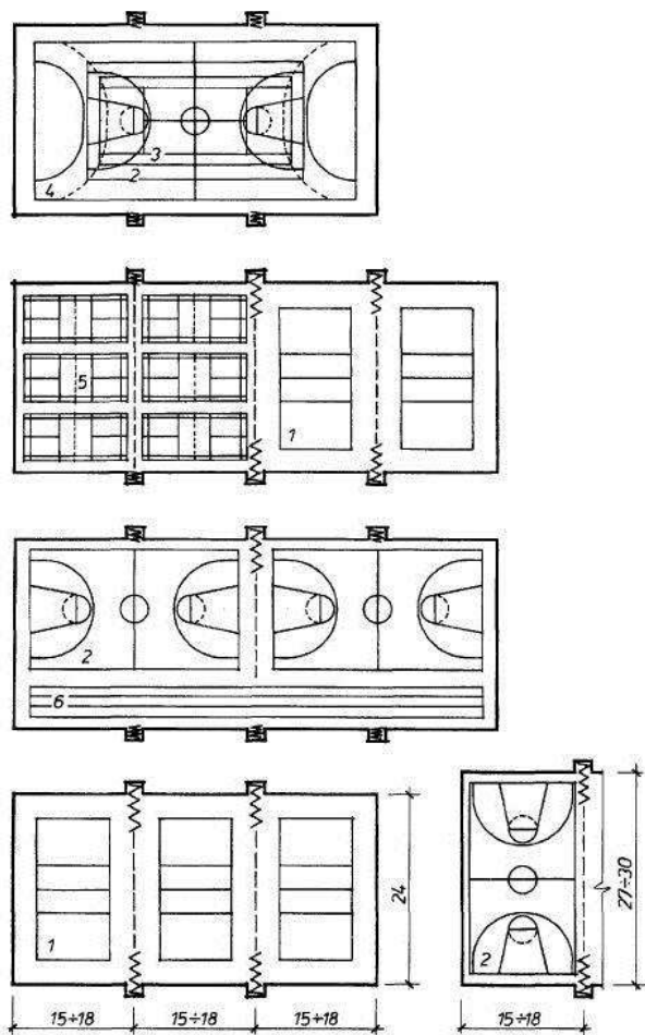
Рис. 17. Схеми трансформації багатофункціональних залів: 1 – майданчик для волейболу, 2 – майданчик для
