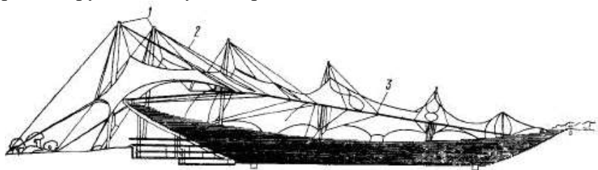
Рис. 15. Дашок вантової конструкції центральної спортивної арени Олімпійського стадіону в Мюнхені: 1 – металеві щогли, 2 – несучі лінви, 3 – стабілізуювальні лінви.
