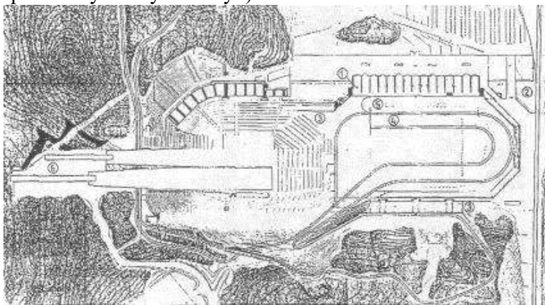
Рис. 21. План лижного стадіону (Лахті, Фінляндія): 1 – допоміжний корпус; 2 – службова зона; 3 – глядацькі трибуни; 4 – місце старту; 5 – місце фінішу; 6 – трампліни для стрибків.
