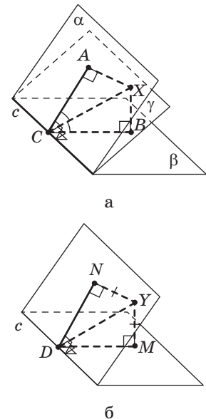
Рис. 299. До доведення теореми про геометричне місце точок, рівновіддалених від граней двогранного кута
