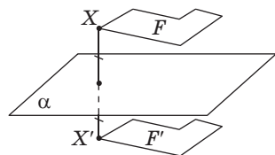
Рис. 234. Фігури F і F' симетричні відносно площини \alpha
