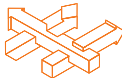
Рис. 100. «Неможливі фігури» О. Рутерсварда
