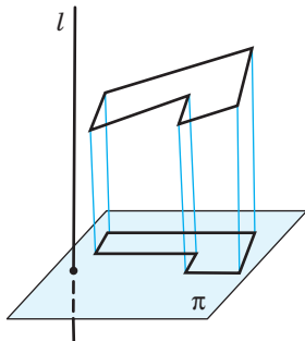
Рис. 197. Ортогональне проєкціювання
