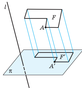
Рис. 83. Паралельне проєкціювання
