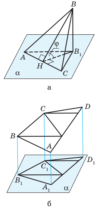
Рис. 199. До доведення формули площі ортогональної проєкції многокутника
