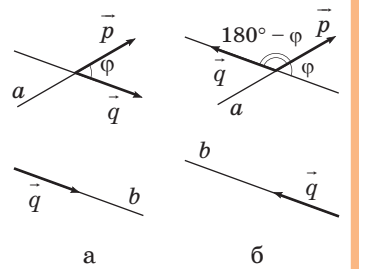
Рис. 281. Визначення кута між прямими в просторі
