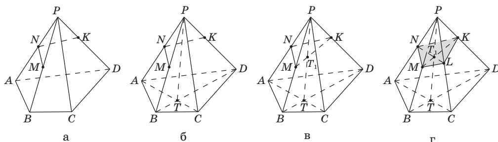
Рис. 105. Побудова перерізу методом проєкцій
