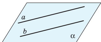
Рис. 39. Паралельні прямі
