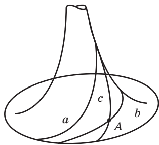
Рис. 16. Псевдосфера
