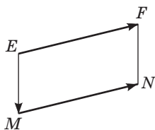
Рис. 251. Рівні вектори
