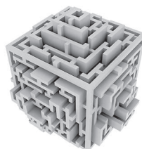
Рис. 45. 3D-лабіринт
