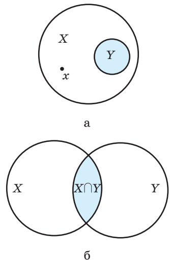
Рис. 27. Особливості вживання символів, пов'язаних із множинами
