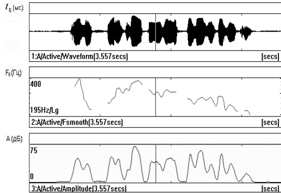
Fig. 1.12. The computer intonogram of the Ukrainian declarative phrase “Треба не розвіяти його як полону за вітром.” (the speaker – Ukrainian woman, UW3)
