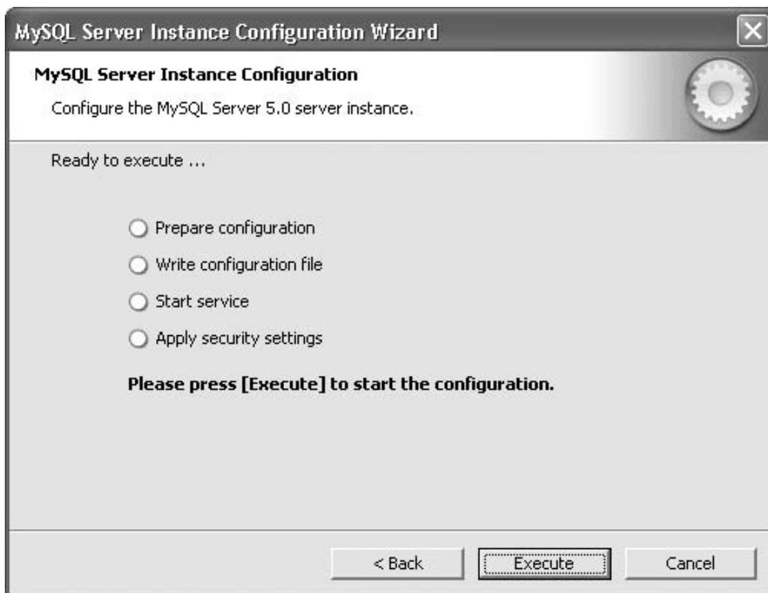
Рис. 1.18. Конфигурирование MySQL
