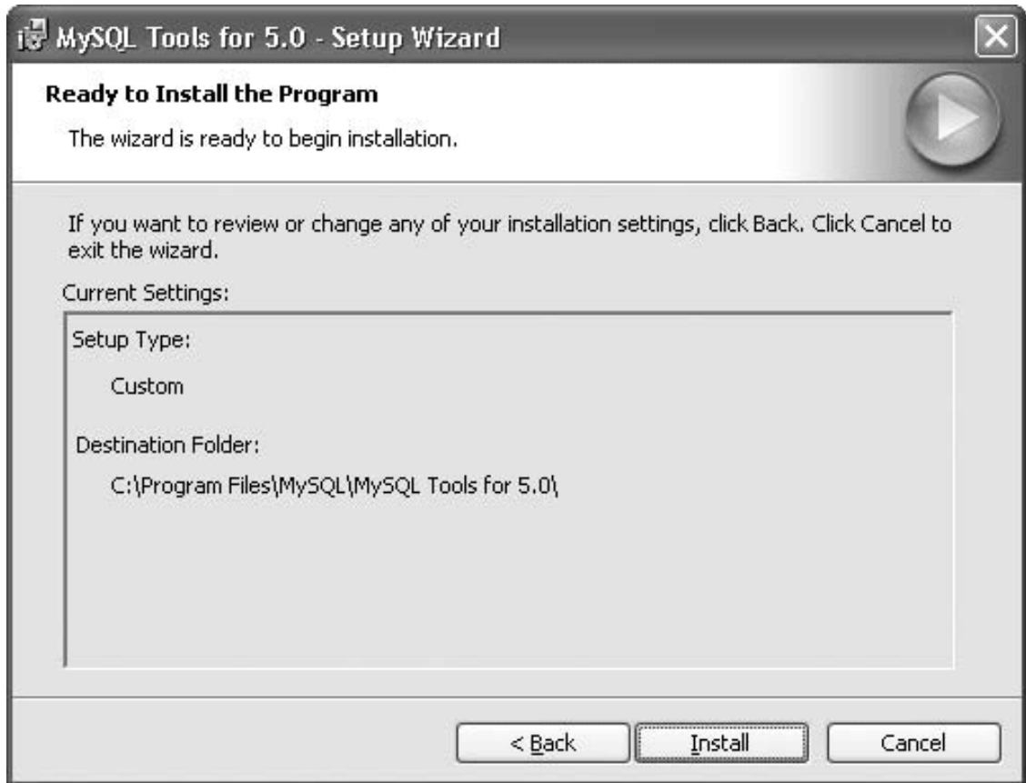
Рис. 1.24. Подтверждение параметров
