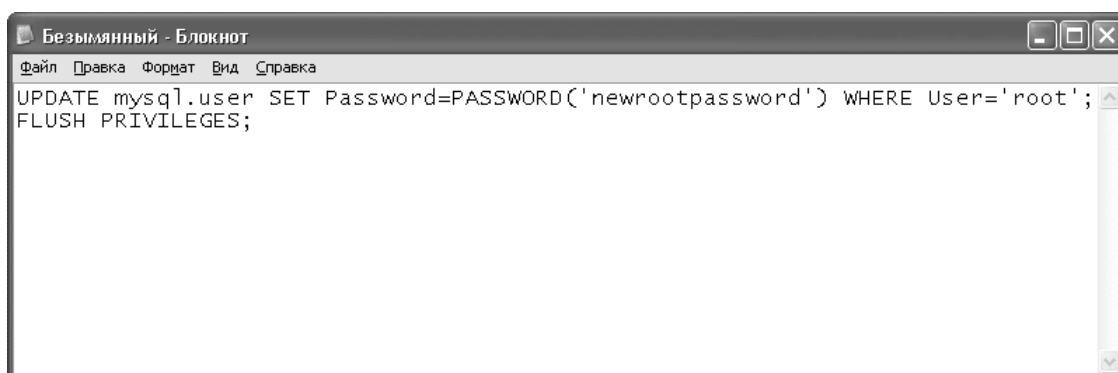
Рис. 5.1. Init-файл
