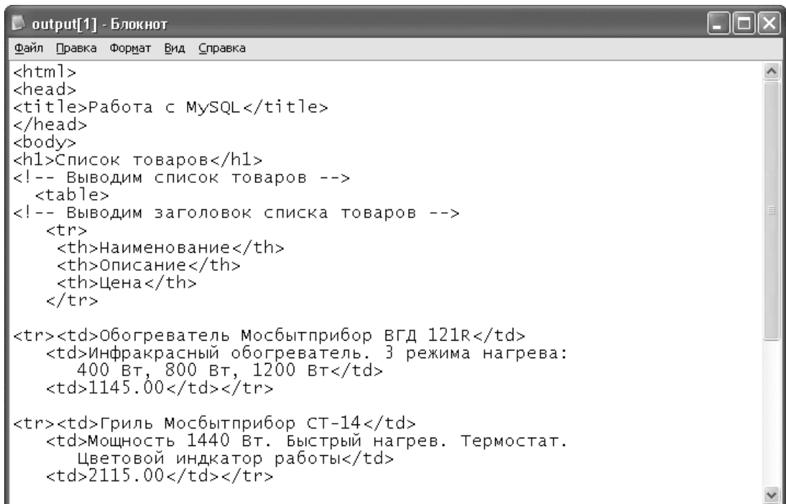
Рис. 4.12. HTML-код страницы
