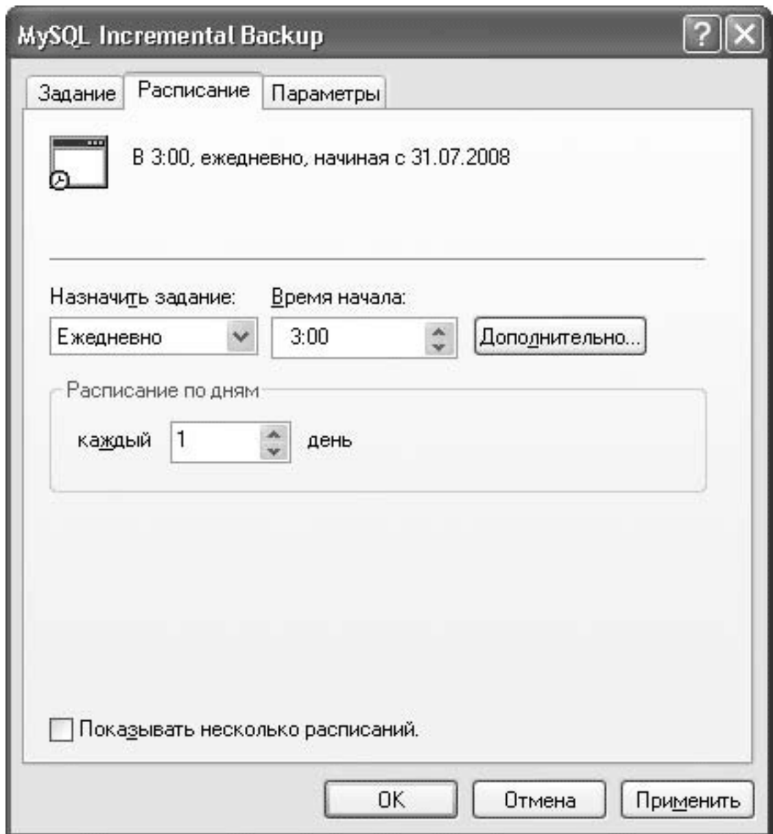
Рис. 5.13. Настройка расписания
