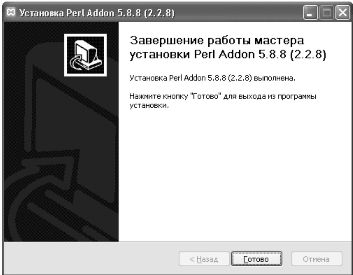
Рис. 4.18. Завершение установки
