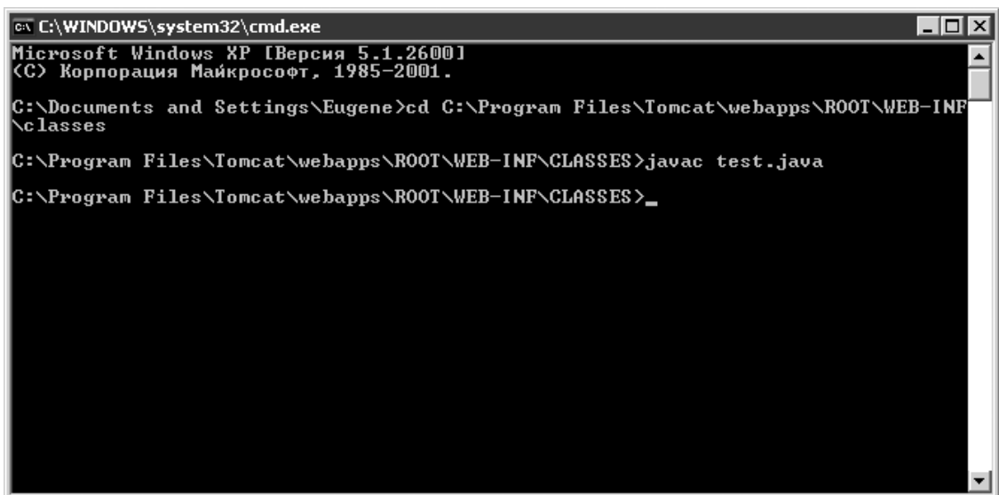
Рис. 4.32. Компиляция сервлета
