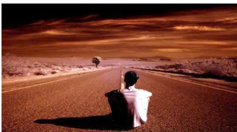
Рис. 8.2. Способи дисоціації
