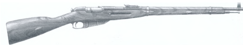
◀ 7,62 мм гвинтівка системи С. Мосіна зр. 1891/1930 рр. Вага: 4 кг. Довжина: 1320 мм. Ємність магазину: 5 набоїв. Скорострільність: 10 постр./хв. Прицільна дальність: 2000 м.
