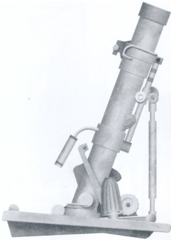
▲ 50-мм німецький міномет зр. 36. Вага: 14 кг. Довжина: 2200 мм. Ємність магазину: 5 набоїв. Скорострільність: 20 постр./хв. Дальність стрільби: 520 м. Вага міни: 0,9 кг.
