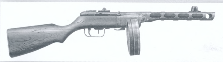
◀ 7,92 мм пістолет-кулемет ППШ-41. Вага: 5,3 кг. Довжина: 842 мм. Ємність магазину: 71 або 35 набоїв. Скорострільність: до 100 постр./хв. Прицільна дальність: 100 – 200, 500 м.
