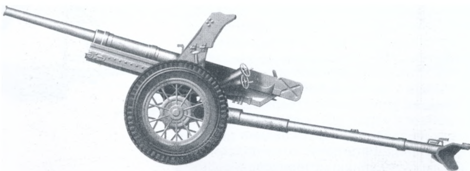
► 45 мм протитанкова гармата зр. 1937 р. Вага: 560 кг у бойовому положенні, 1200 кг — у похідному. Скорострільність: 15–20 постр./хв. Дальність прямого пострілу: 850 м.
