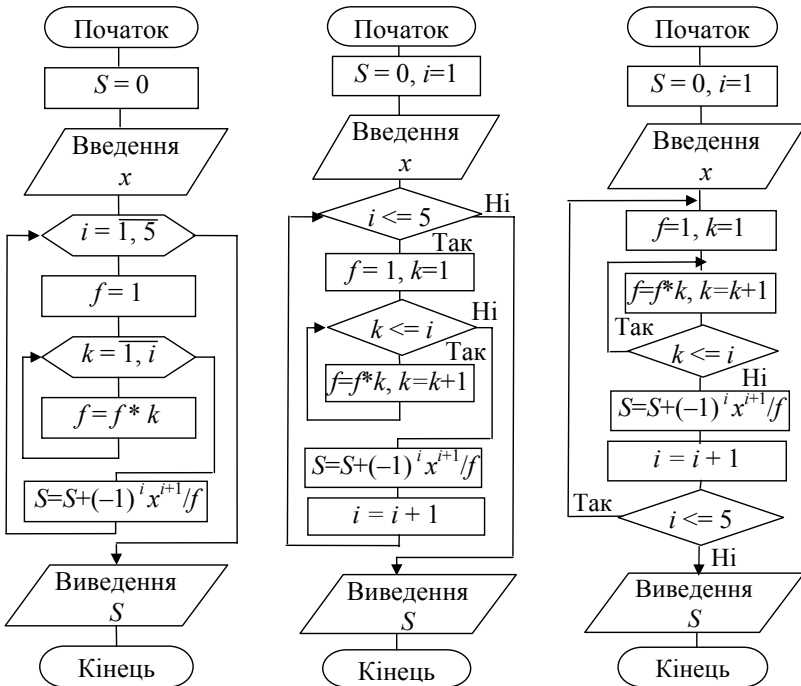
Схеми алгоритмів програм з різними операторами циклу: а – for; б – while; в – do-while
