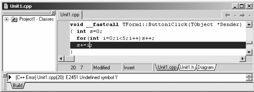
Рис. 14.8. Помилка E2451: змінну s оголошено в іншій області видимості
