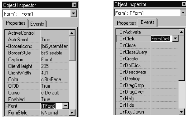
а б Рис. 2.5. Вікна інспектора об'єктів:
