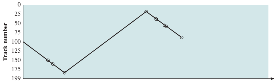
(d) C-SCAN
