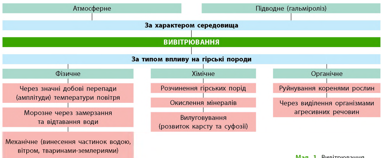
Мал. 1. Вивітрювання.
