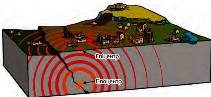
Мал. 1. Схема землетрусу.
