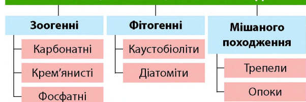
Мал. 1. Гірські породи органічного походження.
